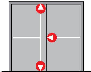
1 bod horizontální uzamykání 2 body vertikální uzamykání Je nutné použít koordinátory zavírání!
