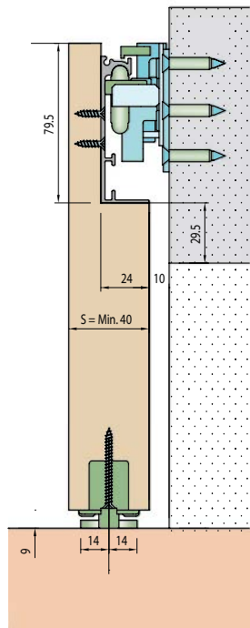
Montáž do stěny
