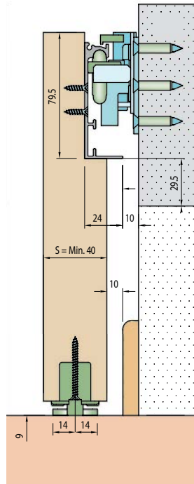
Montáž do stěny + prahová lišta
