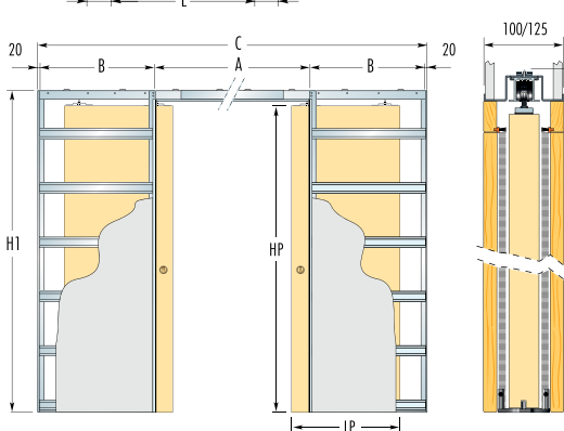
Tabulka rozměrů pro dvoukřídlové provedení Tabulka rozmerov pre dvojkrídlové prevedenie
